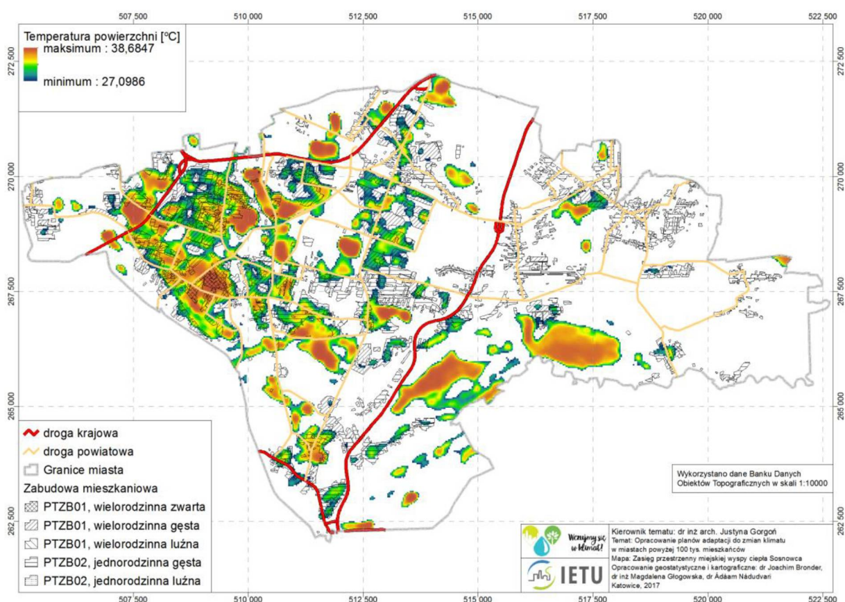
Ryc. 4. Zasięg miejskiej wyspy ciepła w Sosnowcu
